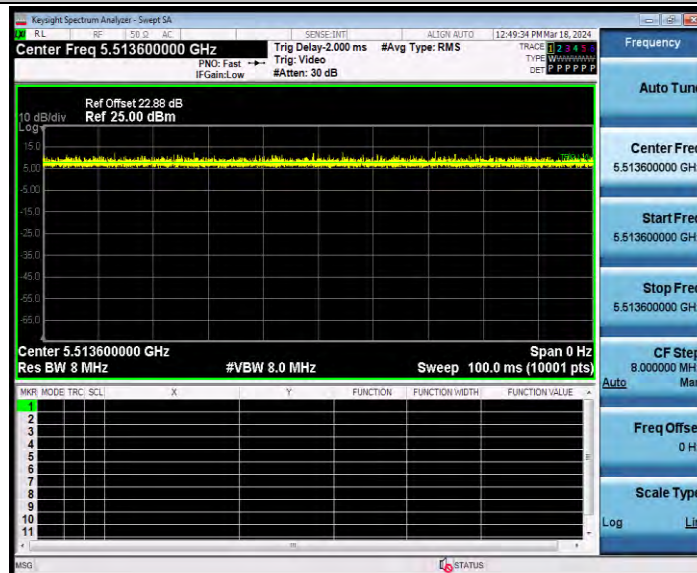
11AX40MIMO_Ant2_5510_484Tone_RU65
