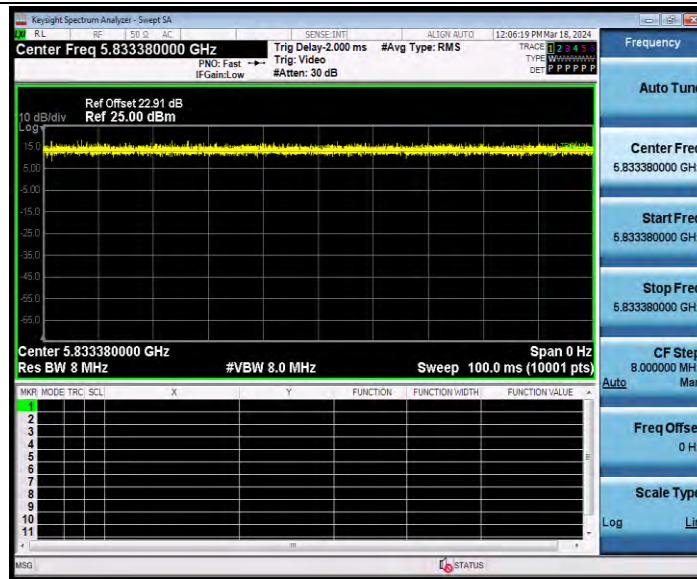
11AX20MIMO_Ant1_5825_52Tone_RU40
