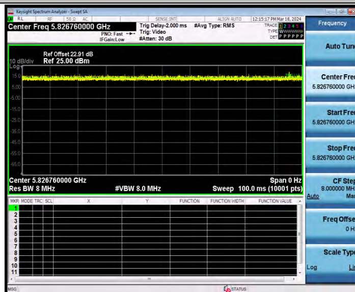
11AX20MIMO_Ant1_5825_106Tone_RU54
