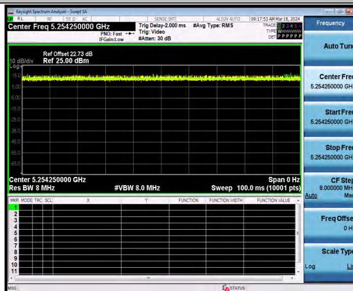
11AX20MIMO_Ant1_5260_52Tone_RU37
