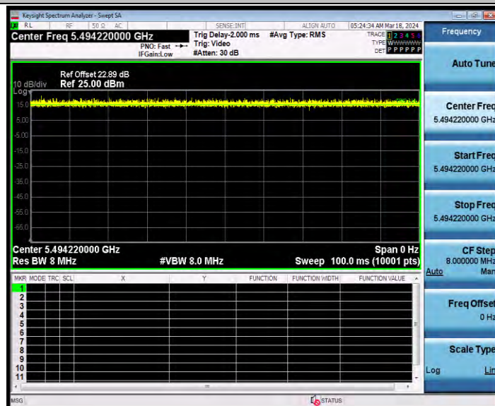
11AX20SISO_Ant2_5500_106Tone_RU53
