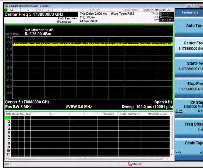
11AX20MIMO_Ant2_5180_26Tone_RU0
