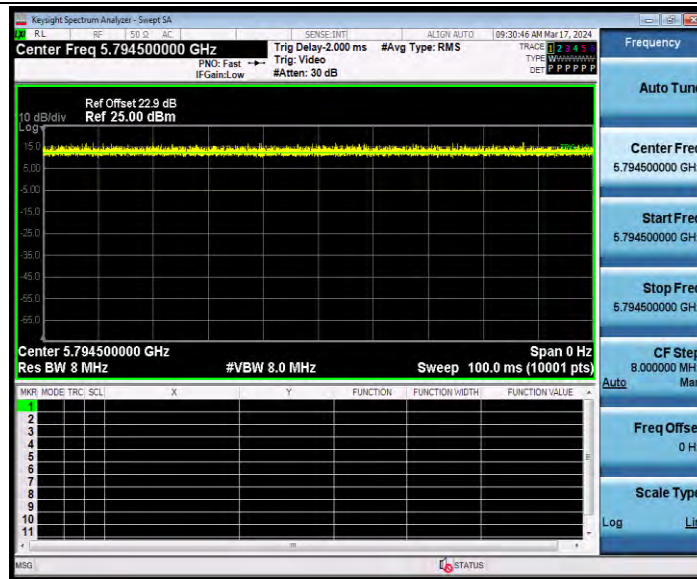
11AX40SISO_Ant2_5795_484Tone_RU65
