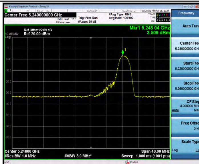
11AX20MIMO_Ant2_5240_26Tone_RU8
