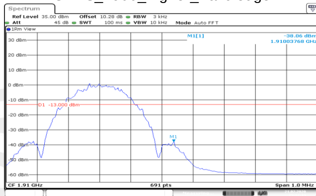
EGPRS_1900(8PSK)_Higher_Band edge
