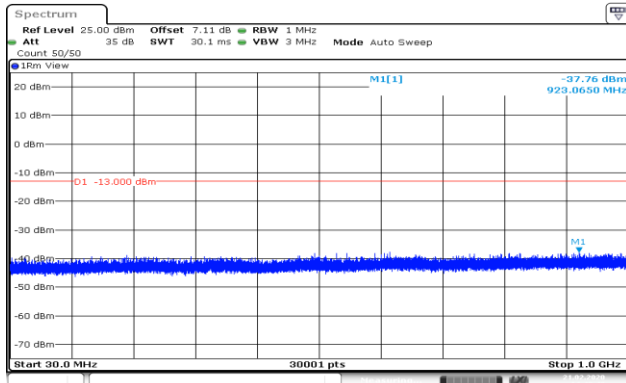
EGPRS_1900(8PSK)_Lower(30MHz-1GHz)
