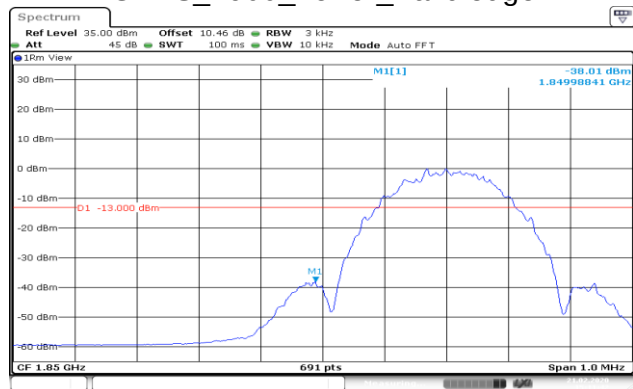
EGPRS_1900(8PSK)_Lower_Band edge
