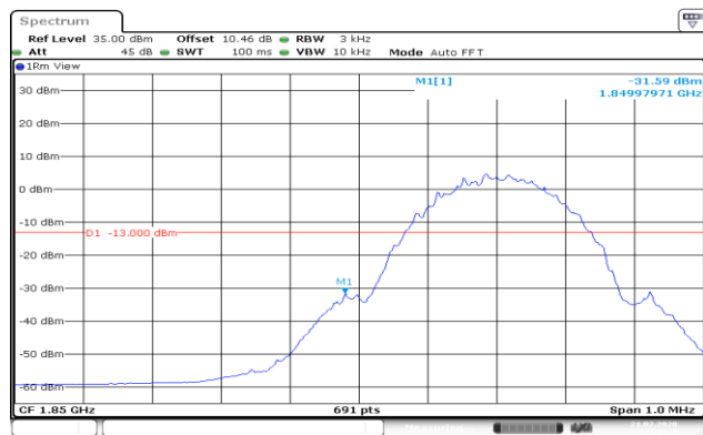
GPRS_1900_Lower_Band edge
