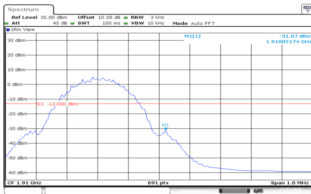
GPRS_1900_Higher_Band edge
