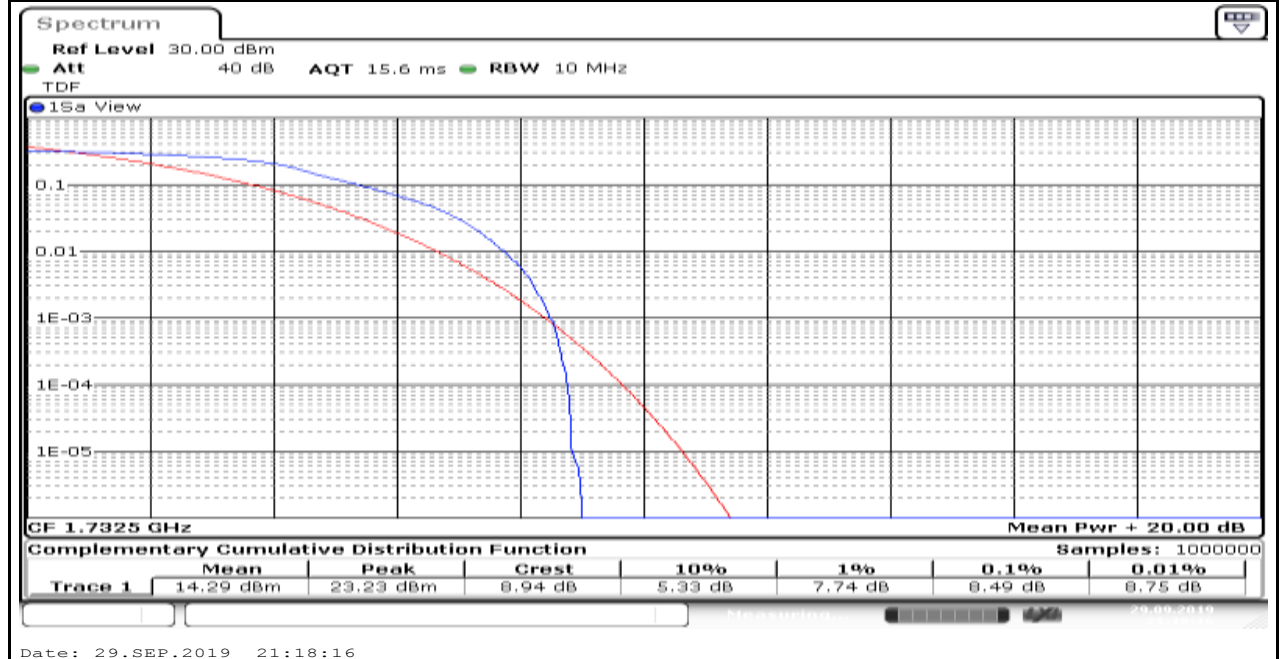
Band4_20MHz_QPSK_20175_6
