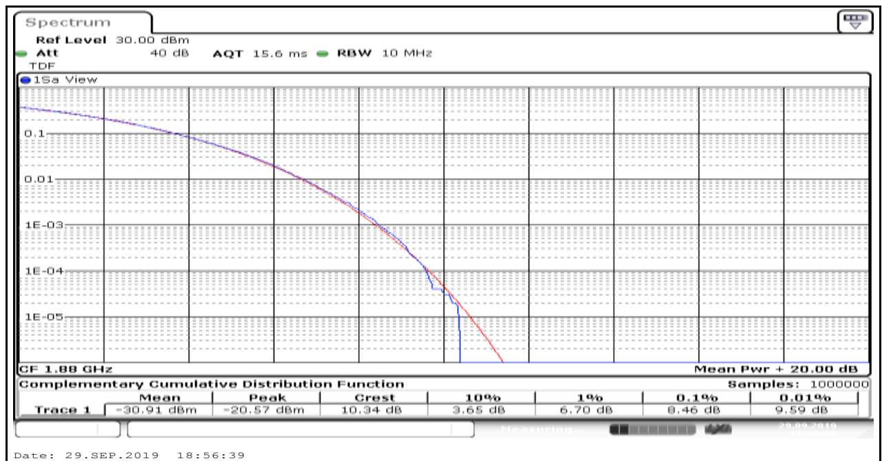
Band2_15MHz_QPSK_18900_6
