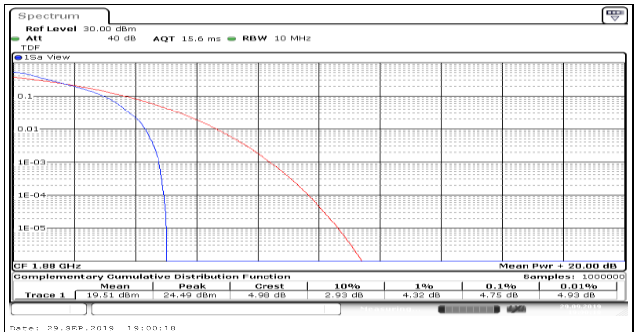
Band2_20MHz_QPSK_18900_6
