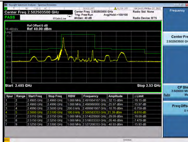
Band7-10MHz-QPSK-20800-50RB#0
