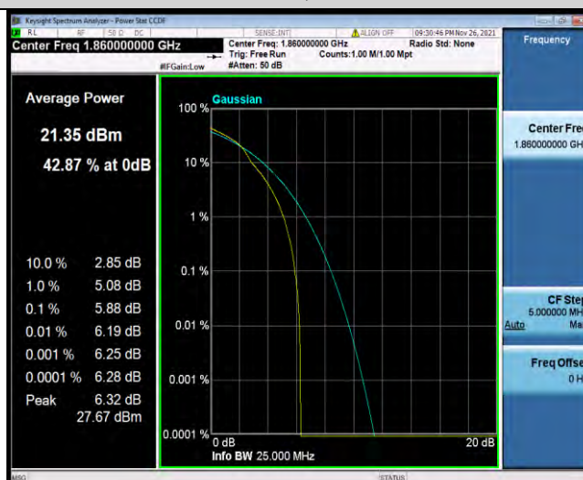
Band2-20MHz-16QAM-18700-27RB#0
