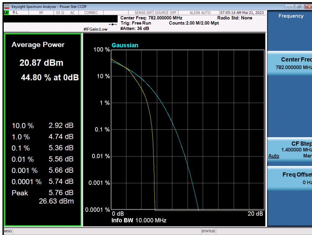
Plot 7-107. PAR Plot (LTE Band 13 - 10MHz 16-QAM - 27 RB)
