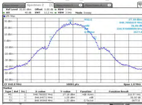
26dB BW_GSM_850_EGPRS_848.8
