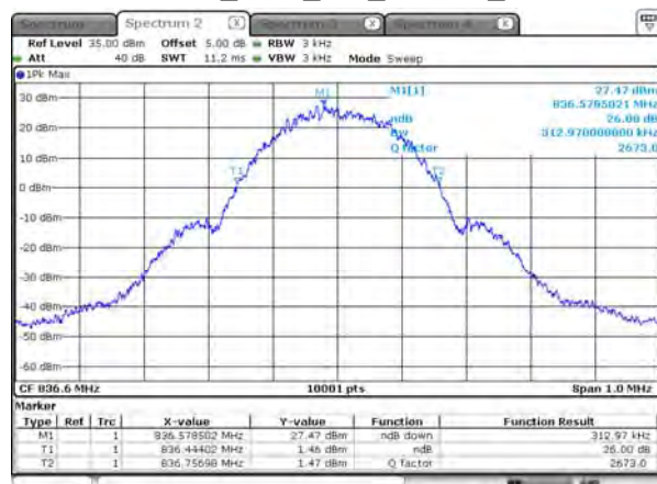
26dB BW_GSM_850_EGPRS_836.6
