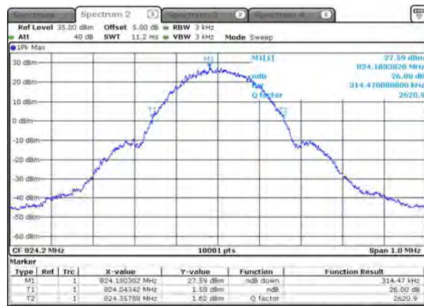
26dB BW_GSM_850_EGPRS_824.2
