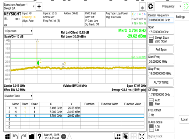
Band77-Part27_10MHz_DFT_s_OFDM_SCS30kHz_BPSK_RB1_1_CH633334_below 18G
