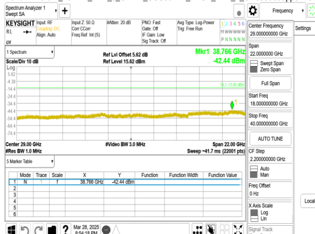
Band77-Part27_20MHz_DFT_s_OFDM_SCS30kHz_BPSK_RB1_1_CH636000upper 18G
