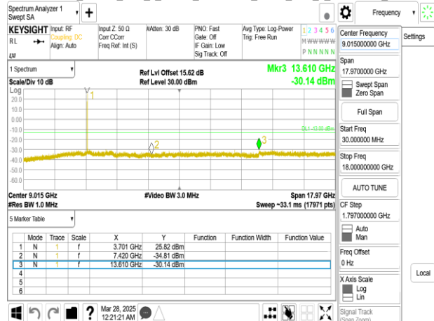
Band77-Part27_20MHz_DFT_s_OFDM_SCS30kHz_BPSK_RB1_1_CH647334upper 18G
