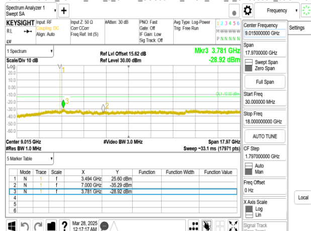
Band77-Part27_15MHz_DFT_s_OFDM_SCS30kHz_BPSK_RB1_1_CH633334_below 18G
