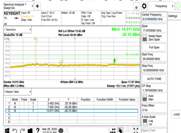
Band77-Part27_20MHz_DFT_s_OFDM_SCS30kHz_BPSK_RB1_1_CH633334_below 18G
