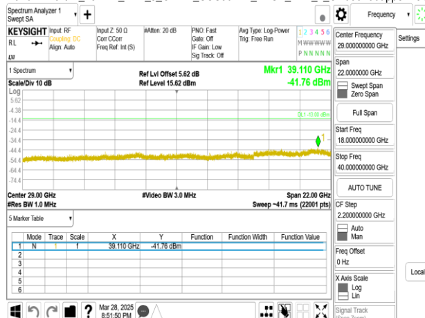
Band77-Part27_15MHz_DFT_s_OFDM_SCS30kHz_BPSK_RB1_1_CH636166upper 18G
