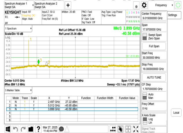
Band41_20MHz_DFT_s_OFDM_SCS30kHz_BPSK_RB1_1_CH501204upper 18G
