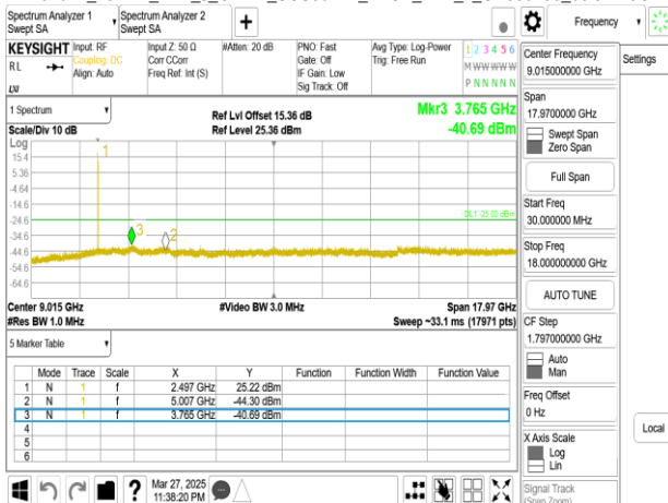
Band41_15MHz_DFT_s_OFDM_SCS30kHz_BPSK_RB1_1_CH500700upper 18G
