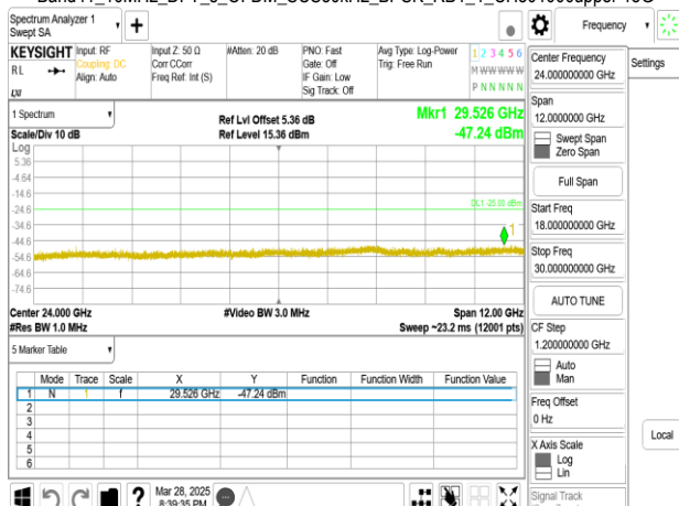
Band41_10MHz_DFT_s_OFDM_SCS30kHz_BPSK_RB1_1_CH501000upper 18G
