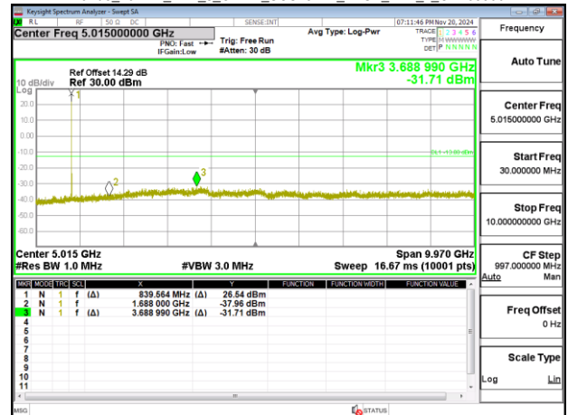
Band5_10MHz_DFT_s_OFDM_SCS15kHz_BPSK_RB1_1_CH168800
