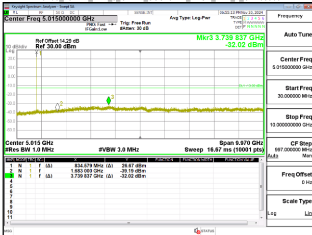
Band5_15MHz_DFT_s_OFDM_SCS15kHz_BPSK_RB1_1_CH168300
