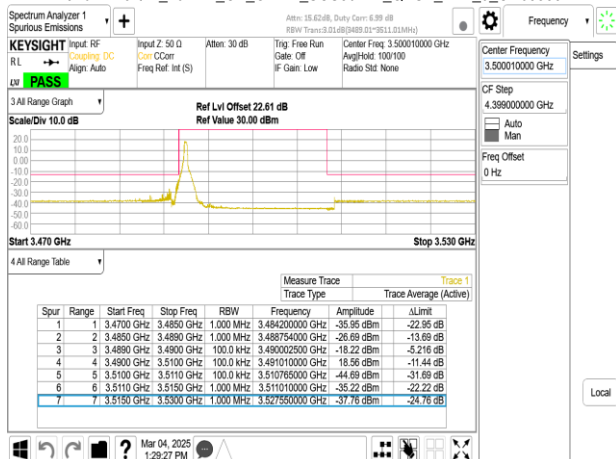
Band77-Part27_20MHz_CP_OFDM_SCS30kHz_QPSK_RB1_0_CH633334
