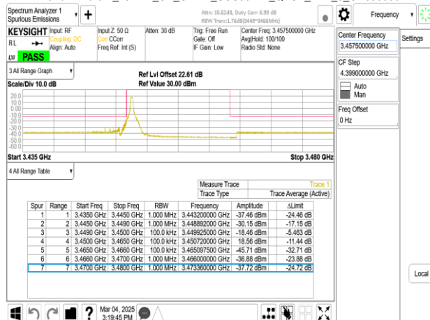
Band77-Part27_15MHz_CP_OFDM_SCS30kHz_QPSK_RB1_0_CH630500
