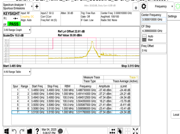
Band77-Part27_10MHz_CP_OFDM_SCS30kHz_QPSK_RB24_0_CH633334
