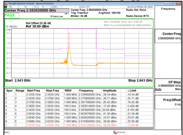
Band41_20MHz_CP_OFDM_SCS30kHz_QPSK_RB1_50_CH518604
