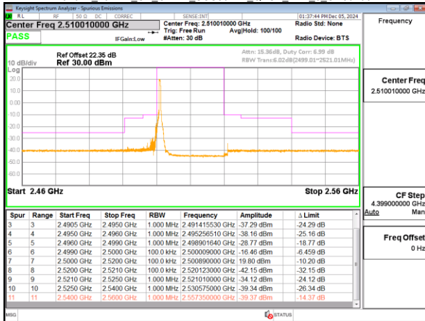
Band41_20MHz_CP_OFDM_SCS30kHz_QPSK_RB1_50_CH502002
