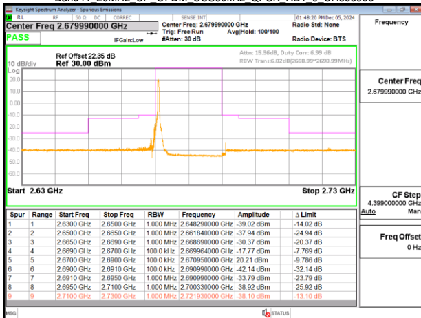
Band41_20MHz_CP_OFDM_SCS30kHz_QPSK_RB1_50_CH535998
