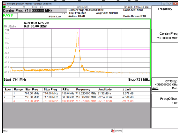
Band12_15MHz_CP_OFDM_SCS15kHz_QPSK_RB1_78_CH141700
