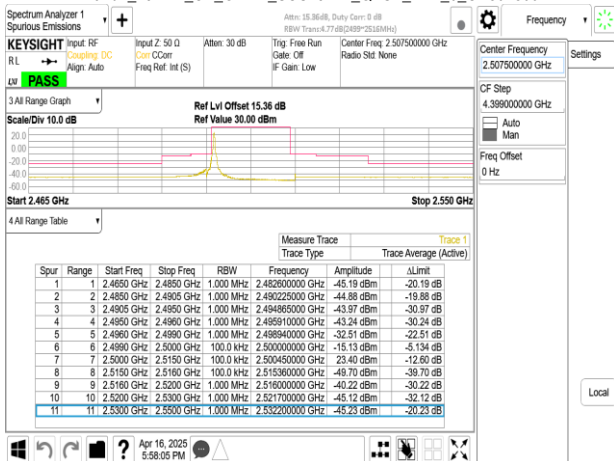
Band7_15MHz_CP_OFDM_SCS15kHz_QPSK_RB1_78_CH501500
