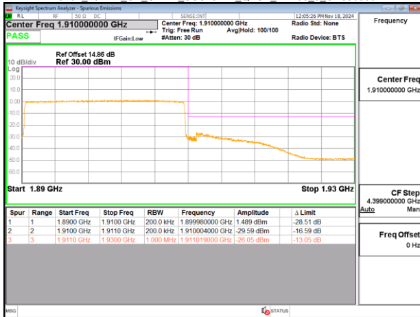
Band2_20MHz_CP_OFDM_SCS15kHz_QPSK_RB1_105_CH380000
