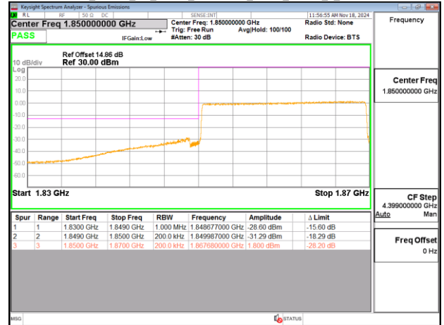
Band2 20MHz CP_OFDM_SCS15kHz QPSK RB1_0_CH372000
