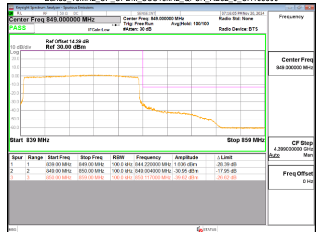
Band5_10MHz_CP_OFDM_SCS15kHz_QPSK_RB52_0_CH168800
