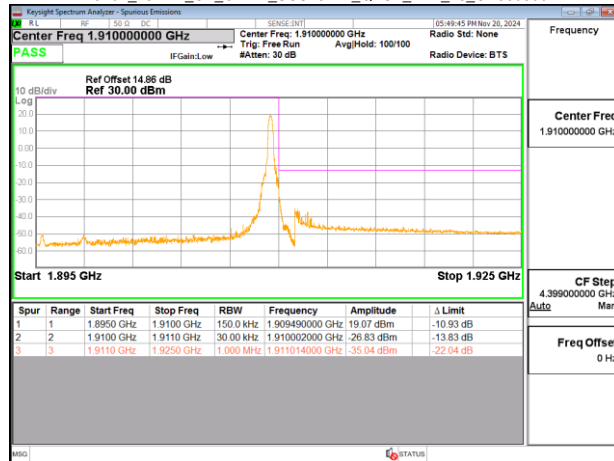
Band2_15MHz CP_OFDM_SCS15kHz QPSK RB79_0_CH380500
