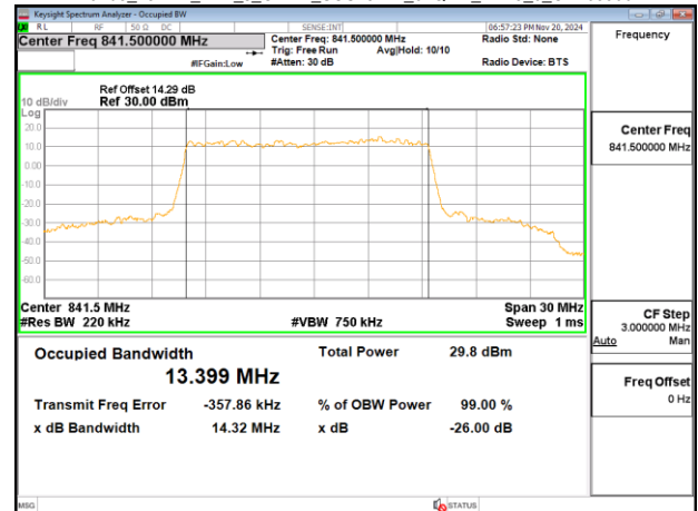
Band5 15MHz DFT_s_OFDM SCS15kHz 64QAM RB75_0 CH168300
