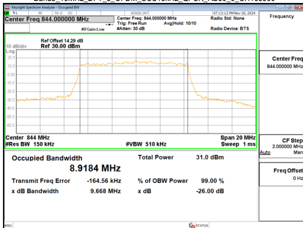
Band5_10MHz_DFT_s_OFDM_SCS15kHz_QPSK_RB50_0_CH168800
