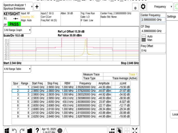
Band38_20MHz_QPSK_RB1_99_CH38000
