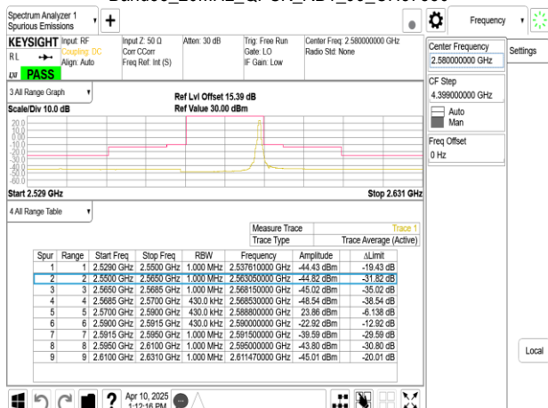
Band38_20MHz_QPSK_RB1_99_CH37850
