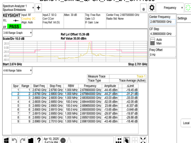
Band41_5MHz_QPSK_RB1_24_CH41565
