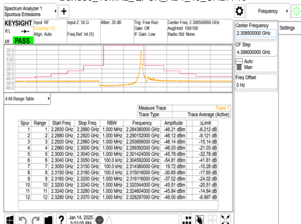
Band30_10MHz_QPSK_RB1_49_CH27710
