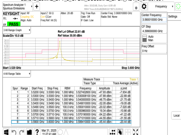
Band48_20MHz_DFT_s_OFDM_SCS30kHz_BPSK_RB1_50_CH673334
