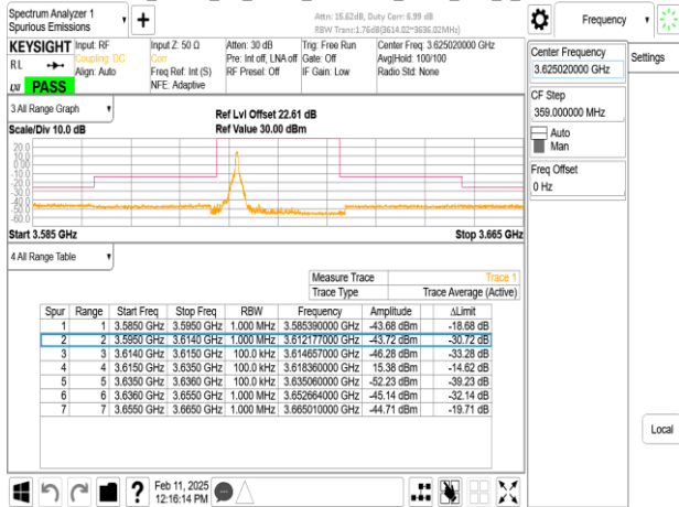
Band48_15MHz_CP_OFDM_SCS30kHz_QPSK_RB1_37_CH641668
