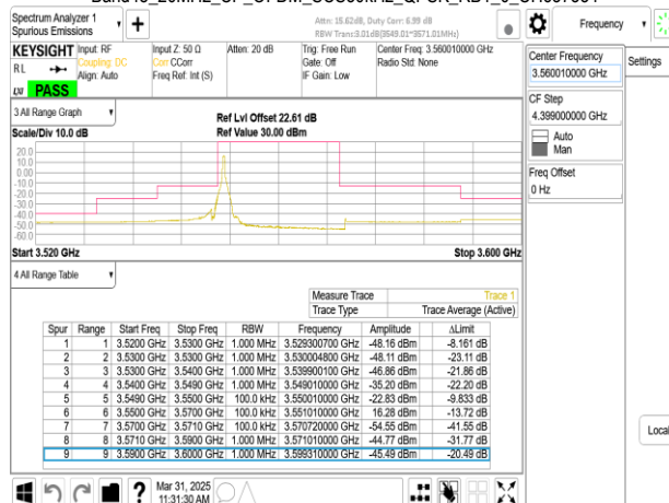
Band48_20MHz_CP_OFDM_SCS30kHz_QPSK_RB1_50_CH637334
