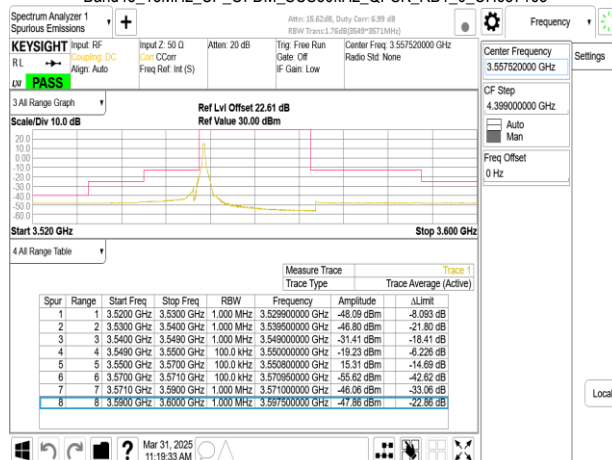
Band48_15MHz_CP_OFDM_SCS30kHz_QPSK_RB1_37_CH637168
