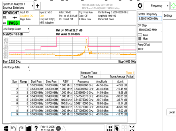
Band48_20MHz_DFT_s_OFDM_SCS30kHz_BPSK_RB50_0_CH673334
