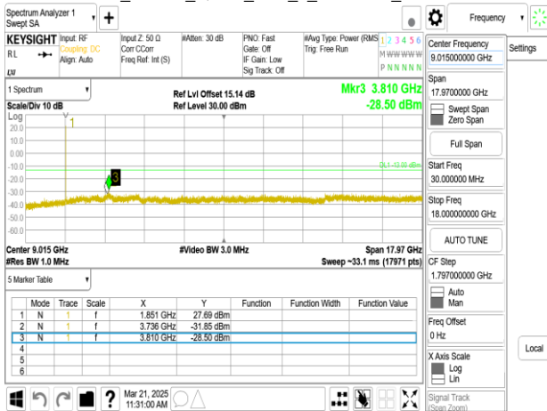
Band2_20MHz_QPSK_RB1_0_CH18700_upper 18G
