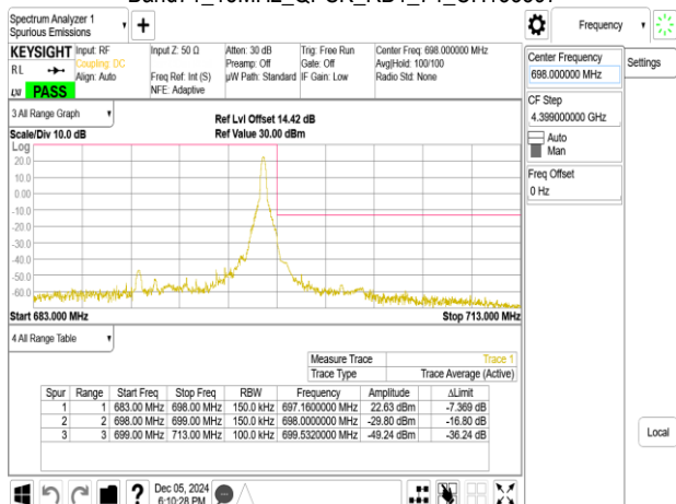
Band71_15MHz_QPSK_RB75_0_CH133397
