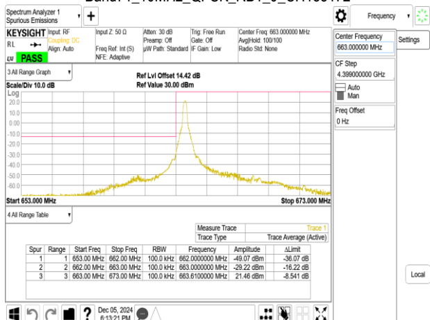
Band71_10MHz_QPSK_RB50_0_CH133172
