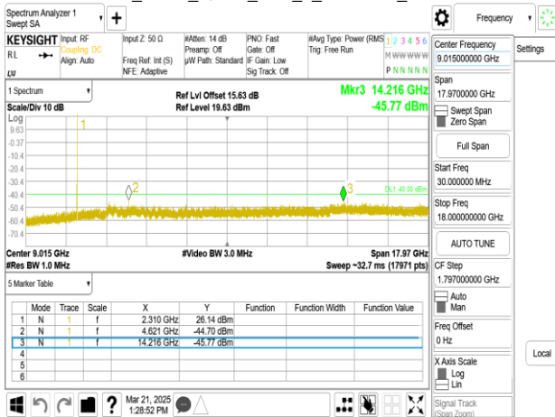
Band30_5MHz_QPSK_RB1_0_CH27735_upper 18G
