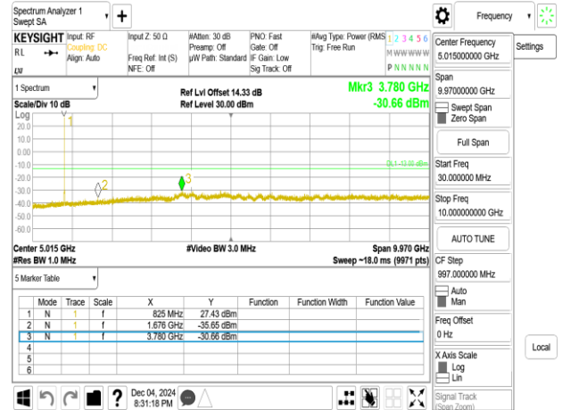
Band5_10MHz_QPSK_RB1_0_CH20525
