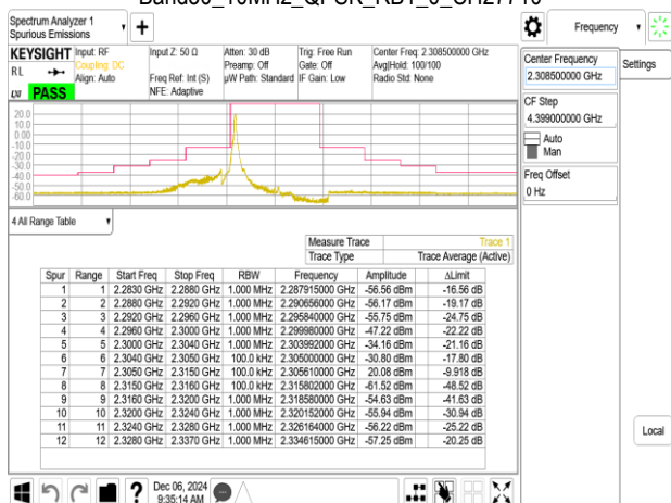
Band30_10MHz_QPSK_RB1_49_CH27710
