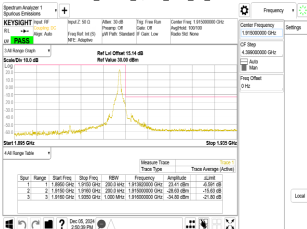
Band25_20MHz_QPSK_RB1_99_CH26590
