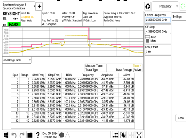
Band30_10MHz_QPSK_RB50_0_CH27710
