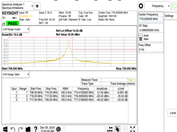
Band17_10MHz_QPSK_RB1_49_CH23800
