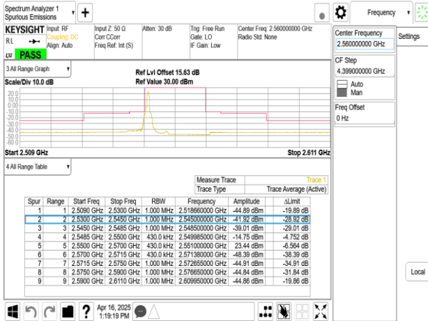
Band7_20MHz_QPSK_RB1_99_CH21350
