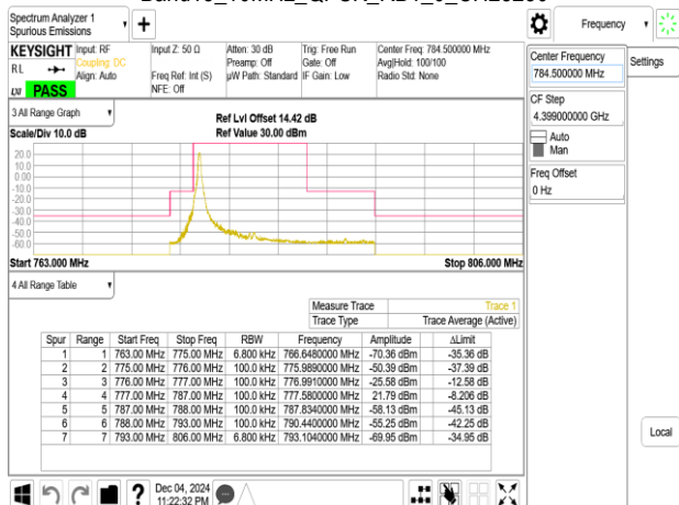
Band13_10MHz_QPSK_RB50_0_CH23230
