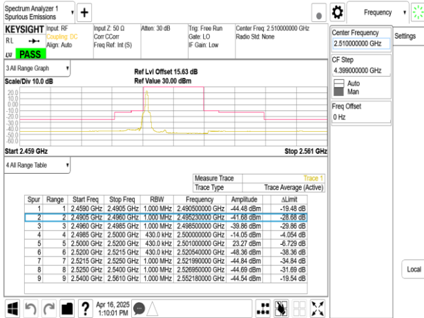
Band7_20MHz_QPSK_RB1_99_CH20850
