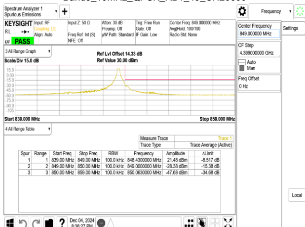
Band5_10MHz_QPSK_RB1_49_CH20600
