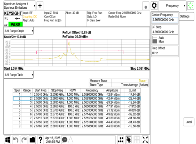
Band7_5MHz_QPSK_RB1_24_CH21425
