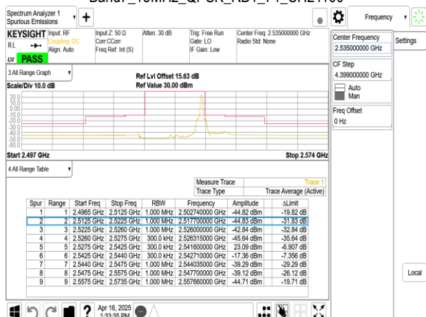
Band7_15MHz_QPSK_RB1_74_CH21100
