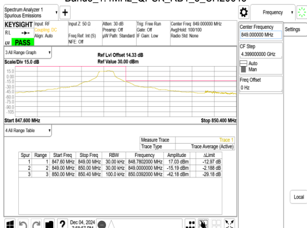
Band5_1.4MHz_QPSK_RB1_5_CH20643
