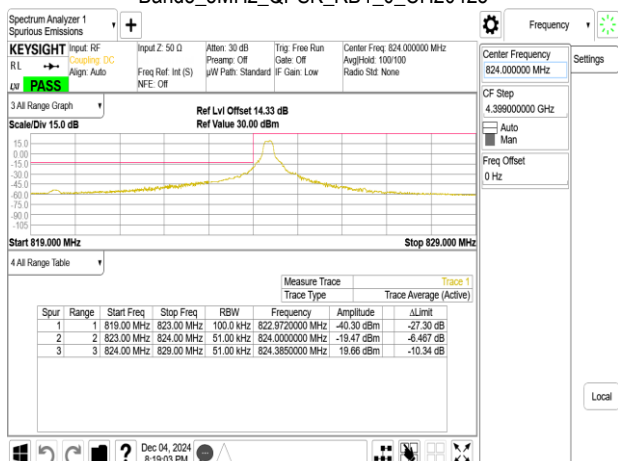
Band5_5MHz_QPSK_RB1_0_CH20425
