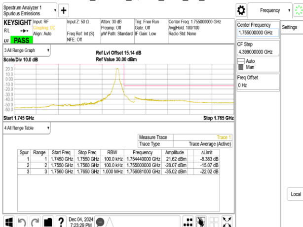
Band4_10MHz_QPSK_RB1_49_CH20350
