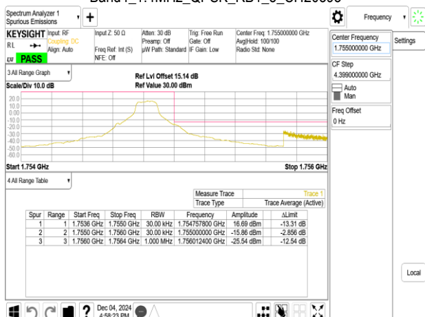
Band4_1.4MHz_QPSK_RB1_5_CH20393
