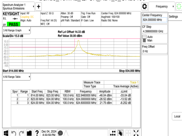
Band5_10MHz_QPSK_RB50_0_CH20450
