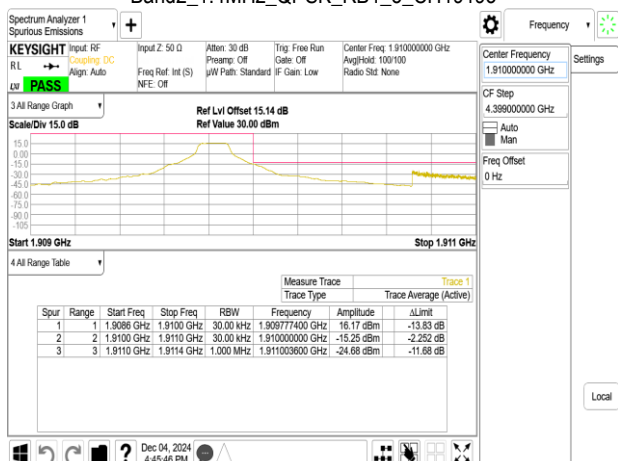
Band2_1.4MHz_QPSK_RB1_5_CH19193
