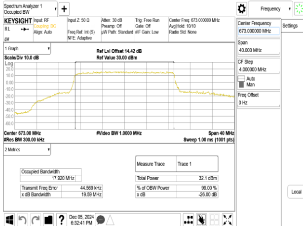
Band71_20MHz_QPSK_RB100_0_CH133222
