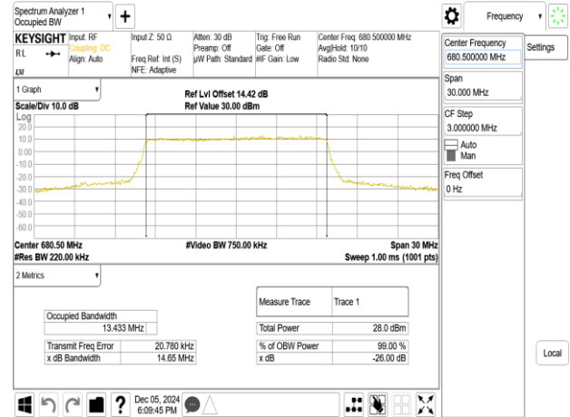
Band71_15MHz_QPSK_RB75_0_CH133397
