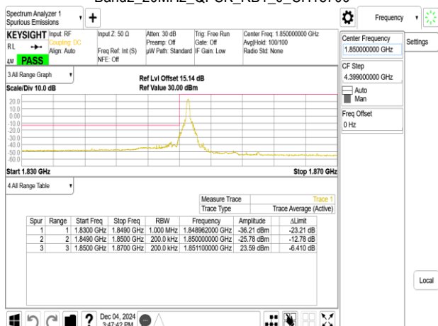
Band2_20MHz_QPSK_RB1_0_CH18700
