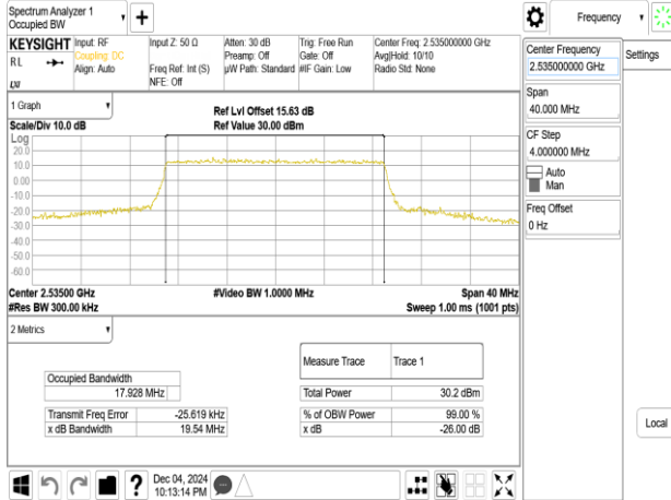
Band7_20MHz_256QAM_RB100_0_CH21100
