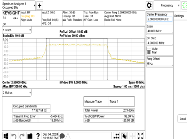
Band7_20MHz_QPSK_RB100_0_CH21350
