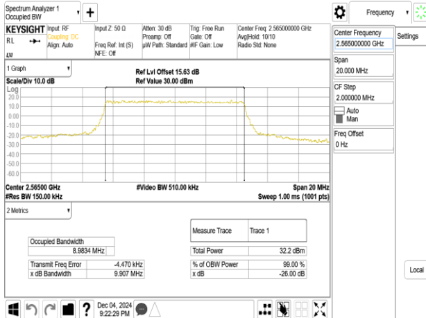
Band7_10MHz_QPSK_RB50_0_CH21400
