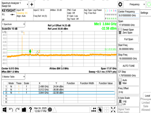
Band41_20MHz_DFT_s_OFDM_SCS30kHz_BPSK_RB1_1_CH501204upper 18G
