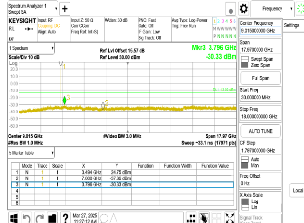
Band77-Part27_15MHz_DFT_s_OFDM_SCS30kHz_BPSK_RB1_1_CH633334_below 18G
