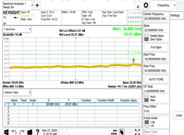
Band77-Part27_15MHz_DFT_s_OFDM_SCS30kHz_BPSK_RB1_1_CH636166upper 18G
