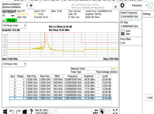
Band77-Part27_15MHz_CP_OFDM_SCS30kHz_QPSK_RB1_37_CH636166
