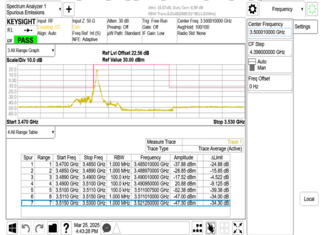
Band77-Part27_20MHz_DFT_s_OFDM_SCS30kHz_BPSK_RB1_50_CH633334
