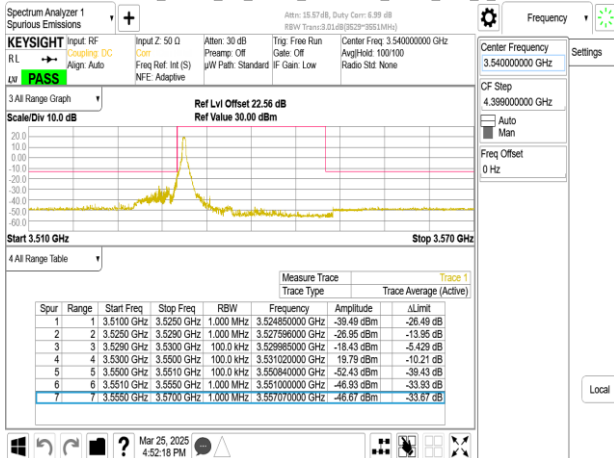
Band77-Part27_20MHz_CP_OFDM_SCS30kHz_QPSK_RB1_50_CH636000
