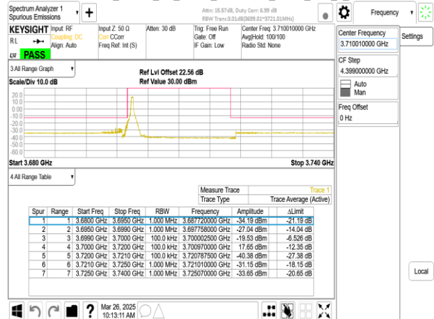
Band77-Part27_20MHz_CP_OFDM_SCS30kHz_QPSK_RB1_50_CH647334
