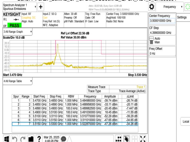
Band77-Part27_20MHz_CP_OFDM_SCS30kHz_QPSK_RB1_50_CH633334
