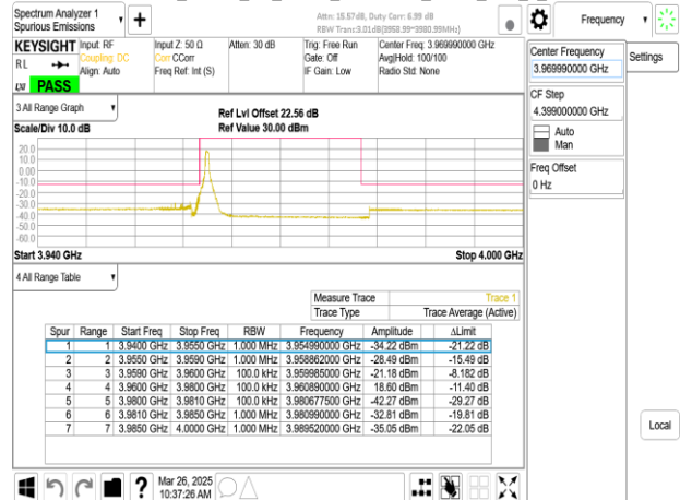
Band77-Part27_20MHz_CP_OFDM_SCS30kHz_QPSK_RB1_50_CH664666
