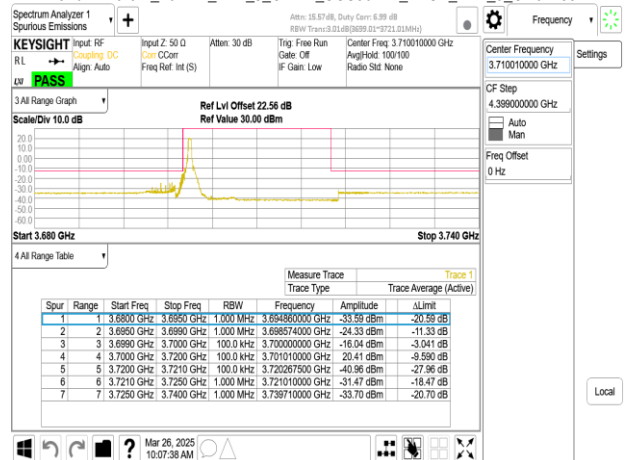
Band77-Part27_20MHz_DFT_s_OFDM_SCS30kHz_BPSK_RB1_50_CH647334
