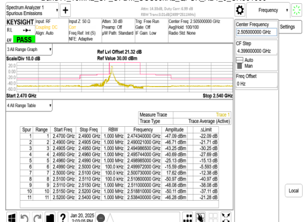
Band41_10MHz_CP_OFDM_SCS30kHz_QPSK_RB1_0_CH501000
