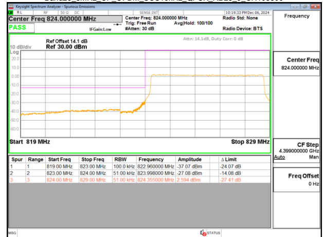
Band26 5MHz CP OFDM SCS15kHz QPSK RB25 0 CH165300
