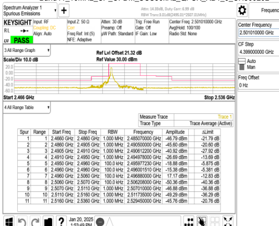
Band41_10MHz_CP_OFDM_SCS30kHz_QPSK_RB1_0_CH500202
