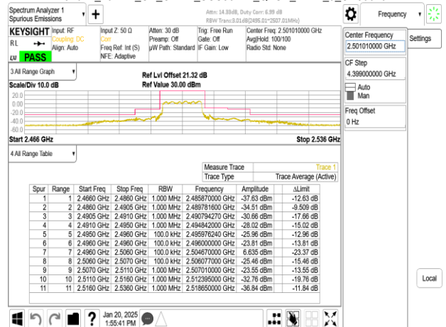
Band41_10MHz_CP_OFDM_SCS30kHz_QPSK_RB1_0_CH501000
