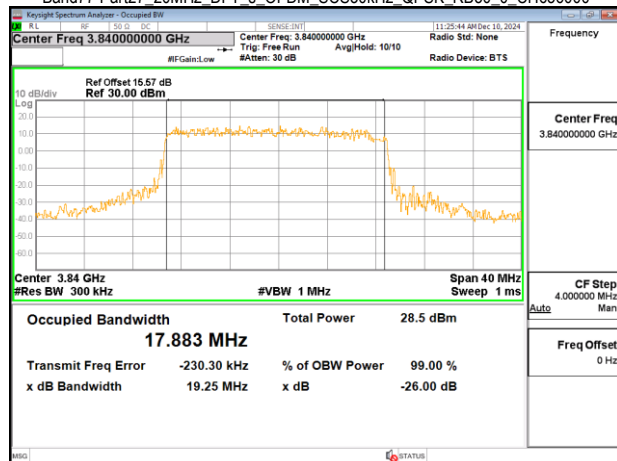
Band77-Part27 20MHz DFT s OFDM SCS30kHz QPSK RB50 0 CH656000
