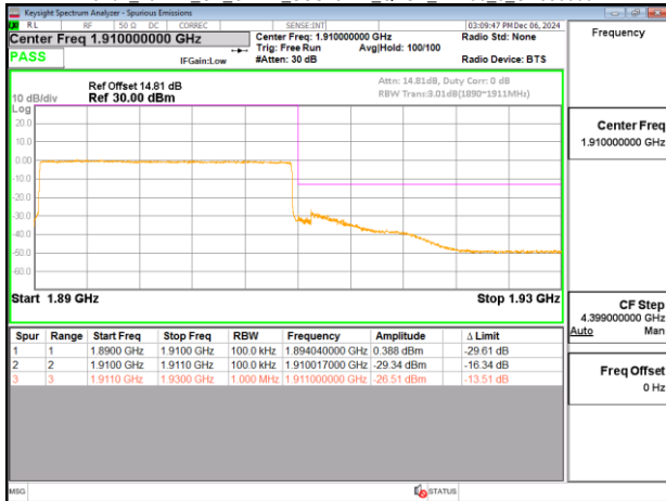
Band2 20MHz CP OFDM SCS15kHz QPSK RB1_105 CH380000
