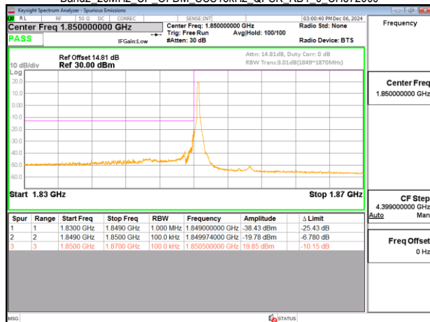
Band2 20MHz CP_OFDM_SCS15kHz QPSK RB1_0 CH372000
