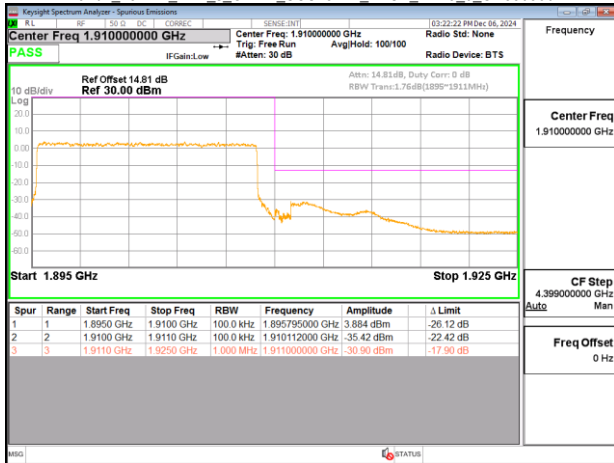
Band2_15MHz CP_OFDM_SCS15kHz QPSK RB1_0_CH371500
