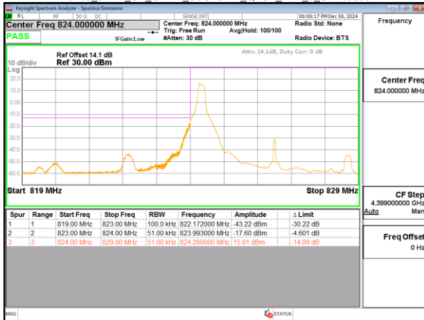
Band5 5MHz CP OFDM SCS15kHz QPSK RB25 0 CH165300
