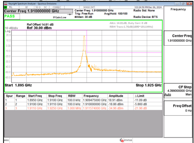
Band2_15MHz CP_OFDM_SCS15kHz QPSK RB79_0_CH380500
