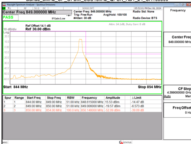
Band5 5MHz CP OFDM SCS15kHz QPSK RB1 24 CH169300
