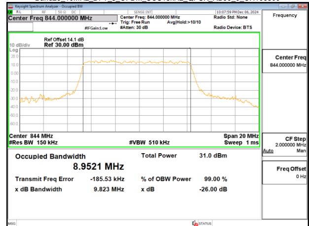
Band26_10MHz DFT s_OFDM_SCS15kHz QPSK RB50_0 CH168800
