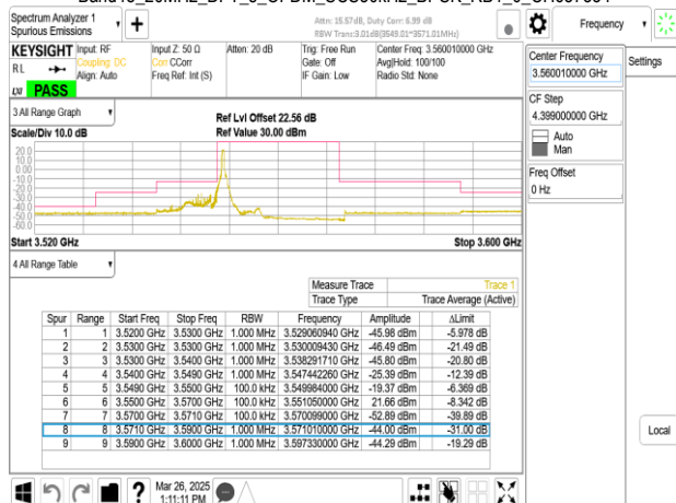
Band48_20MHz_DFT_s_OFDM_SCS30kHz_BPSK_RB1_50_CH637334
