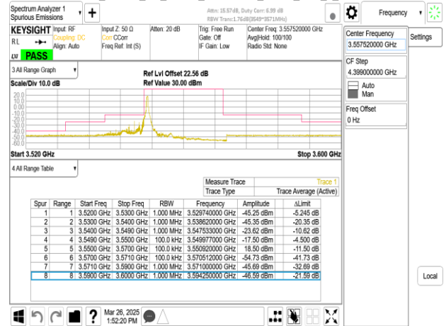
Band48_15MHz_CP_OFDM_SCS30kHz_QPSK_RB1_37_CH637168
