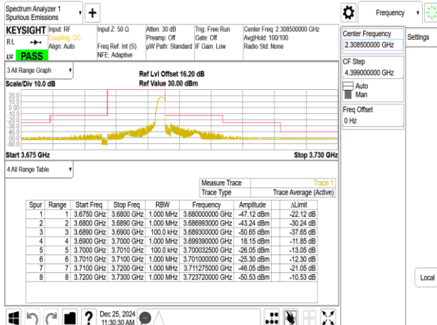
Emission Mask_Band48_10MHz_QPSK_RB1_49_CH56690
