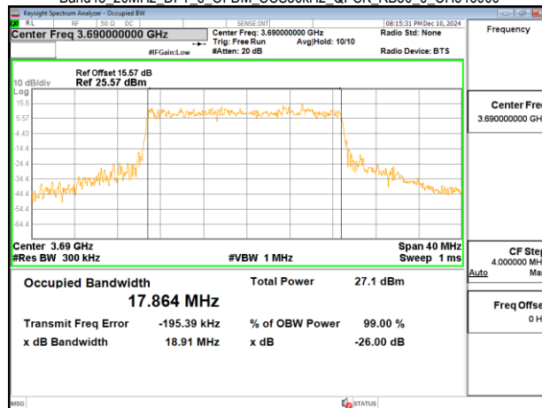
Band48 20MHz DFT s OFDM SCS30kHz QPSK RB50_0 CH646000
