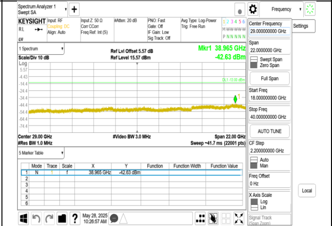
Band77-Part27_10MHz_DFT_s_OFDM_SCS30kHz_BPSK_RB1_1_CH633334_upper 18G
