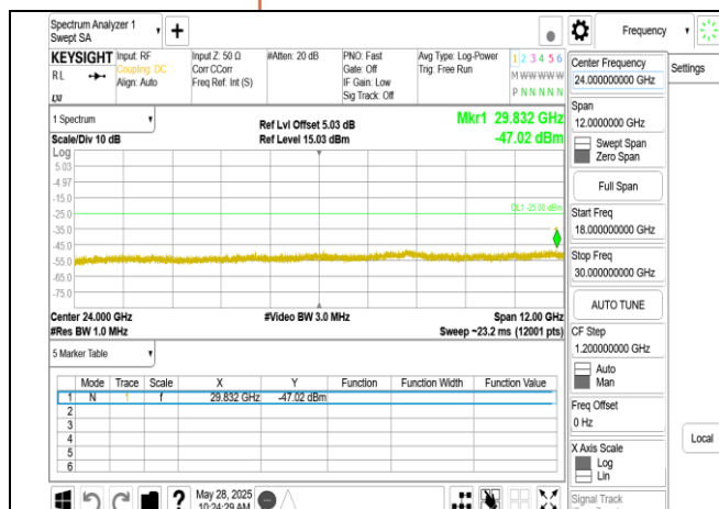
Band41_20MHz_DFT_s_OFDM_SCS30kHz_BPSK_RB1_1_CH501204_upper 18G
