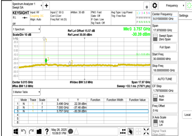
Band77-Part27_10MHz_DFT_s_OFDM_SCS30kHz_BPSK_RB1_1_CH633334_below 18G
