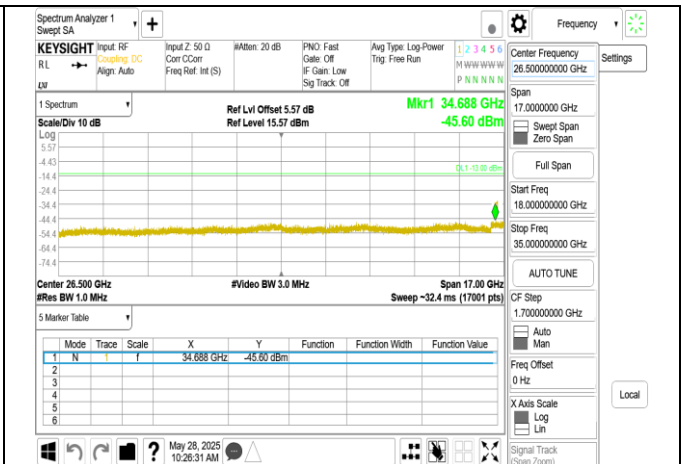
Band77-Part27_10MHz_DFT_s_OFDM_SCS30kHz_BPSK_RB1_1_CH630334_upper 18G
