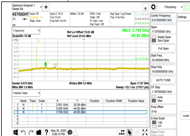
Band7_20MHz_DFT_s_OFDM_SCS15kHz_BPSK_RB1_1_CH502000_below_18G
