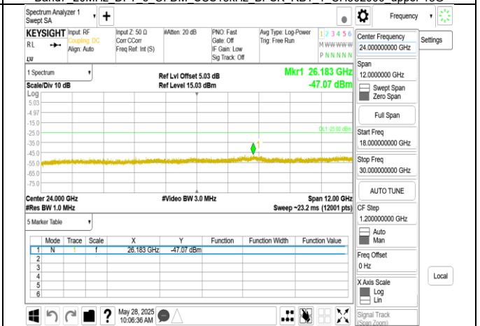
Band7_20MHz_DFT_s_OFDM_SCS15kHz_BPSK_RB1_1_CH507000_upper_18G
