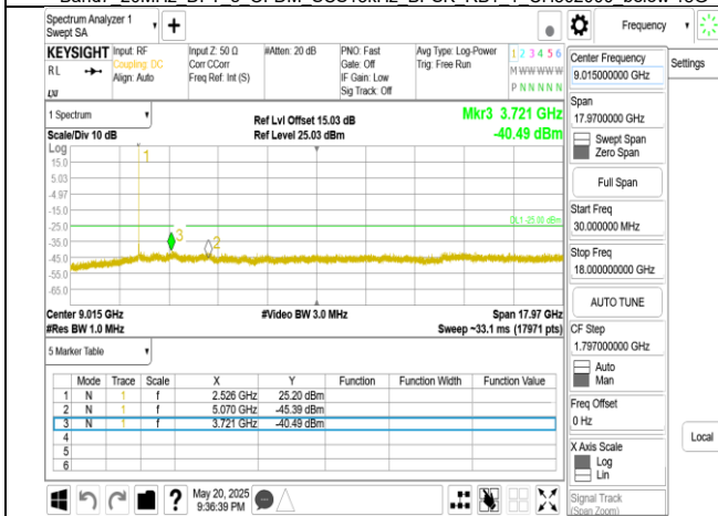
Band7_20MHz_DFT_s_OFDM_SCS15kHz_BPSK_RB1_1_CH507000_below_18G
