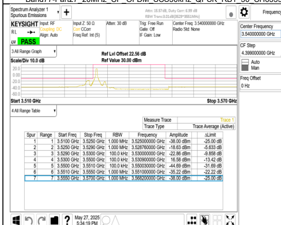
Band77-Part27 20MHz CP OFDM SCS30kHz QPSK RB1_0 CH636000
