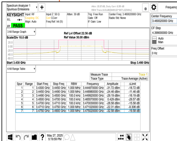
Band77-Part27 20MHz CP OFDM SCS30kHz QPSK RB51_0 CH630668
