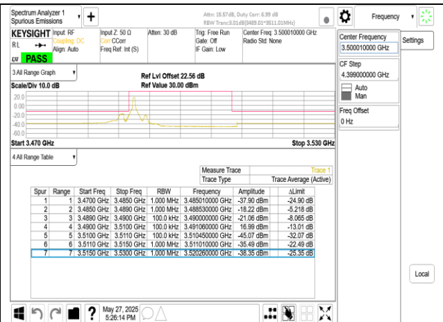
Band77-Part27 20MHz CP OFDM SCS30kHz QPSK RB1_0 CH633334
