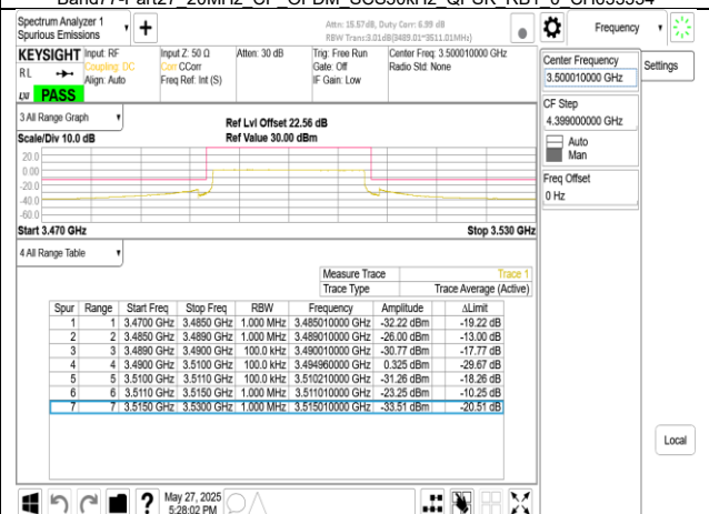
Band77-Part27 20MHz CP OFDM SCS30kHz QPSK RB51_0 CH633334
