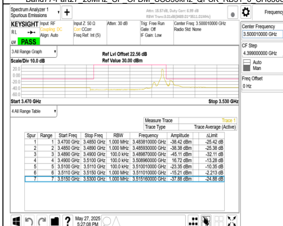
Band77-Part27 20MHz CP OFDM SCS30kHz QPSK RB1_50 CH633334
