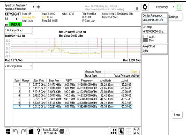
Band77-Part27 15MHz CP OFDM SCS30kHz QPSK RB1_0 CH633334
