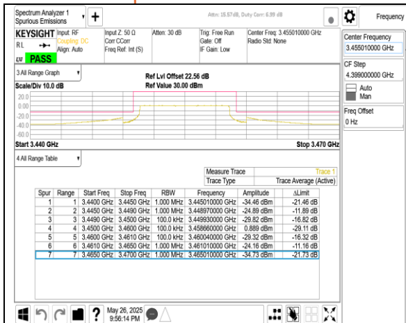
Band77-Part27 10MHz CP OFDM SCS30kHz QPSK RB24_0 CH630334
