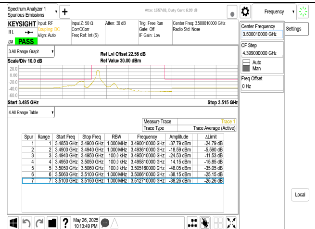
Band77-Part27 10MHz CP OFDM SCS30kHz QPSK RB1_0 CH633334
