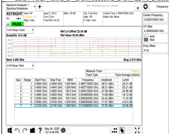
Band77-Part27 10MHz CP OFDM SCS30kHz QPSK RB1_23 CH633334
