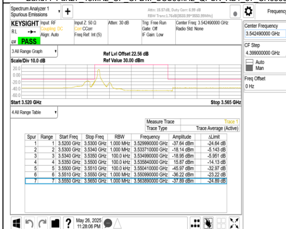
Band77-Part27 15MHz CP OFDM SCS30kHz QPSK RB1_0 CH636166
