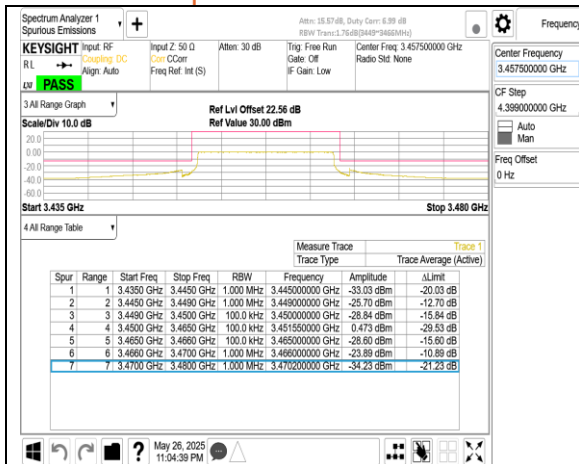
Band77-Part27 15MHz CP OFDM SCS30kHz QPSK RB38_0 CH630500
