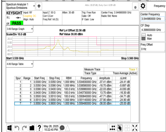
Band77-Part27 10MHz CP OFDM SCS30kHz QPSK RB1_0 CH636332
