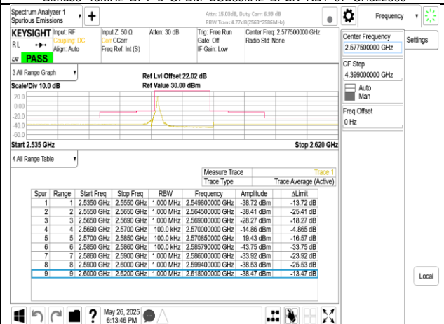
Band38 15MHz CP OFDM SCS30kHz QPSK RB1 0 CH515500
