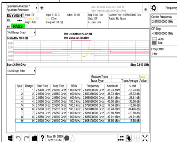
Band38 10MHz CP OFDM SCS30kHz QPSK RB1 23 CH515000
