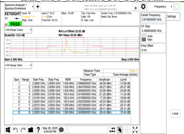
Band38 10MHz CP OFDM SCS30kHz QPSK RB1 0 CH523000
