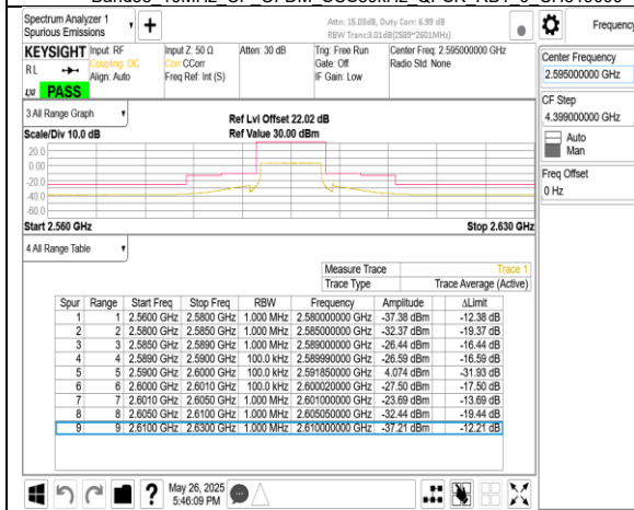
Band38 10MHz CP OFDM SCS30kHz QPSK RB24 0 CH519000
