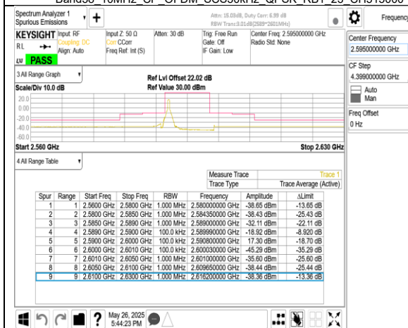
Band38 10MHz CP OFDM SCS30kHz QPSK RB1 0 CH519000
