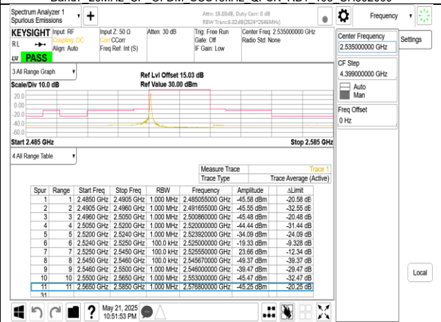
Band7 20MHz CP OFDM SCS15kHz QPSK RB1 0 CH507000
