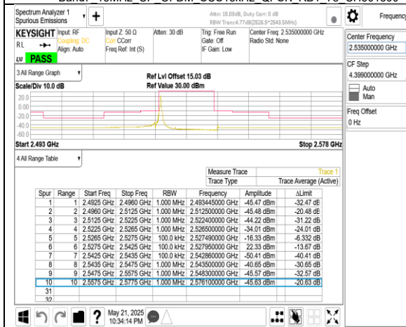
Band7 15MHz CP OFDM SCS15kHz QPSK RB1 0 CH507000
