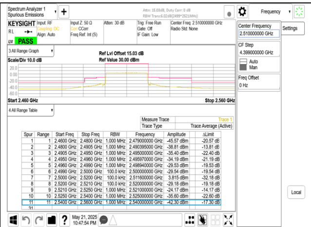
Band7 20MHz CP OFDM SCS15kHz QPSK RB106 0 CH502000
