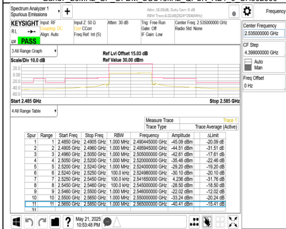
Band7 20MHz CP OFDM SCS15kHz QPSK RB106 0 CH507000
