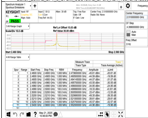
Band7 20MHz CP OFDM SCS15kHz QPSK RB1 0 CH502000
