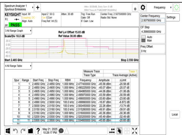
Band7 15MHz CP OFDM SCS15kHz QPSK RB1 0 CH501500
