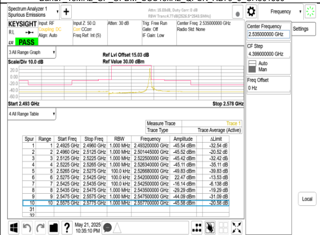
Band7 15MHz CP OFDM SCS15kHz QPSK RB1 78 CH507000
