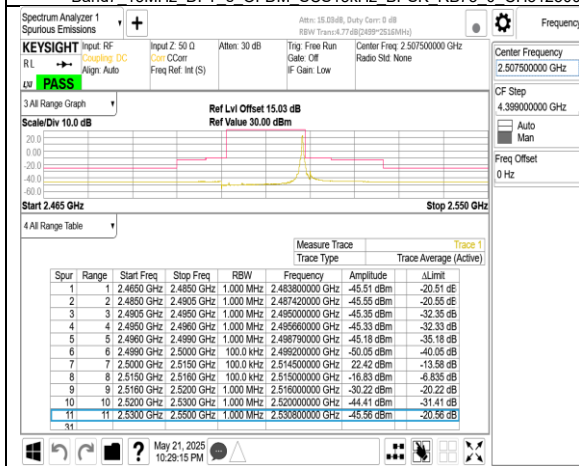
Band7 15MHz CP OFDM SCS15kHz QPSK RB1 78 CH501500
