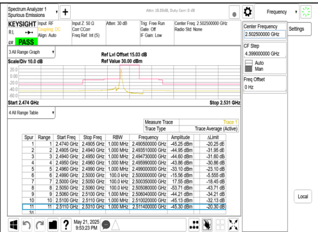
Band7 5MHz CP OFDM SCS15kHz QPSK RB1 0 CH500500
