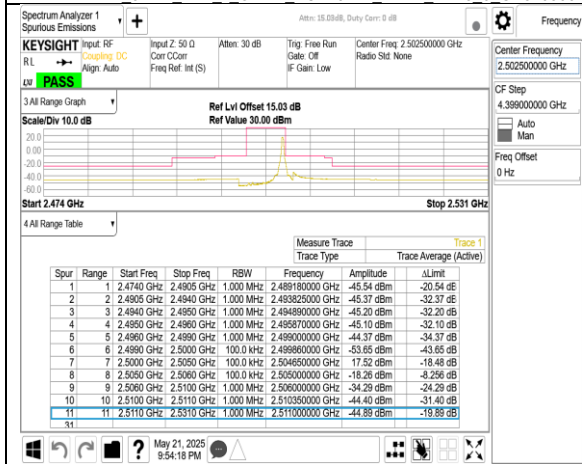
Band7 5MHz CP OFDM SCS15kHz QPSK RB1 24 CH500500
