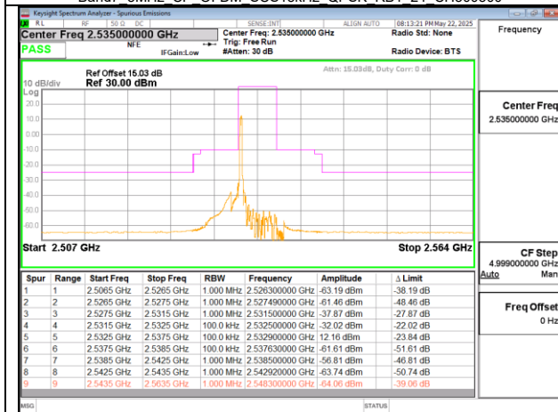
Band7 5MHz CP OFDM SCS15kHz QPSK RB1 0 CH507000
