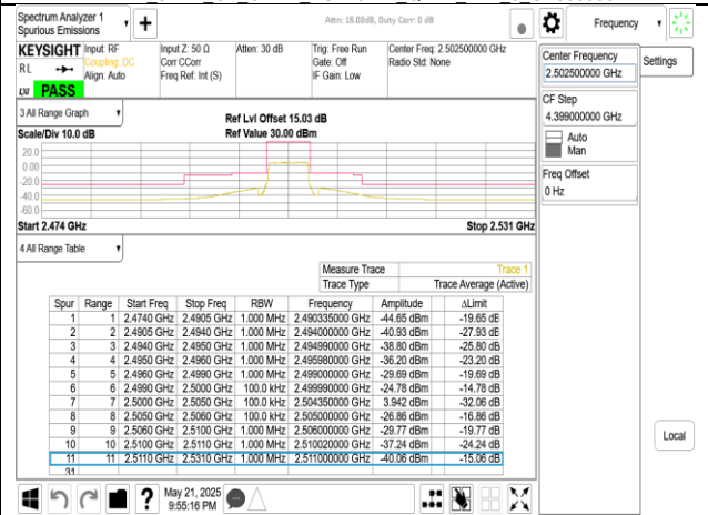
Band7 5MHz CP OFDM SCS15kHz QPSK RB25 0 CH500500
