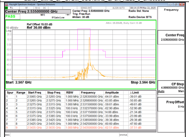
Band7 5MHz CP OFDM SCS15kHz QPSK RB1 24 CH507000
