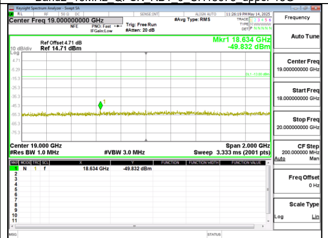
Band2_15MHz_QPSK_RB1_0_CH18900_upper_18G
