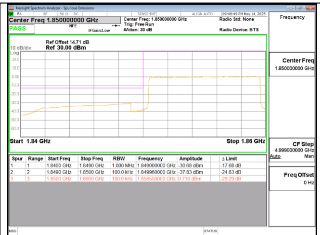
Band2 10MHz QPSK RB50 0 CH18650
