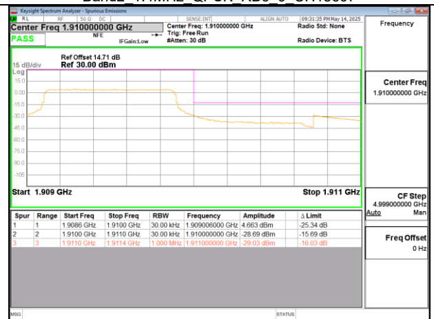
Band2 1.4MHz QPSK RB6 0 CH19193
