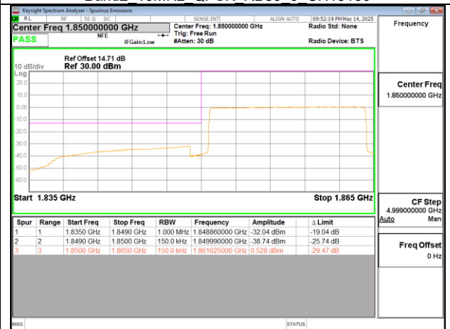
Band2 15MHz QPSK RB75 0 CH18675
