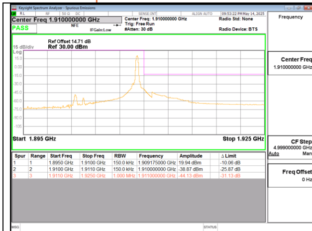
Band2 15MHz QPSK RB1 74 CH19125
