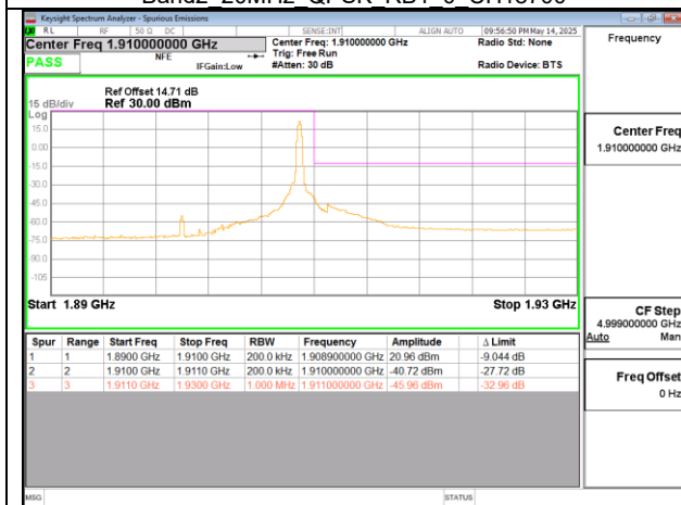
Band2 20MHz QPSK RB1 99 CH19100
