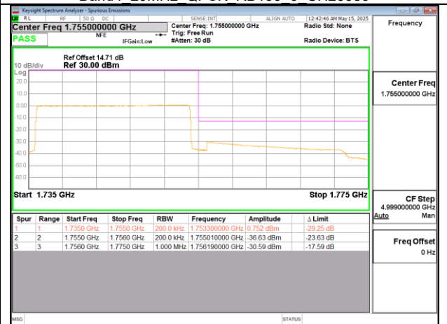
Band4 20MHz QPSK RB100 0 CH20300
