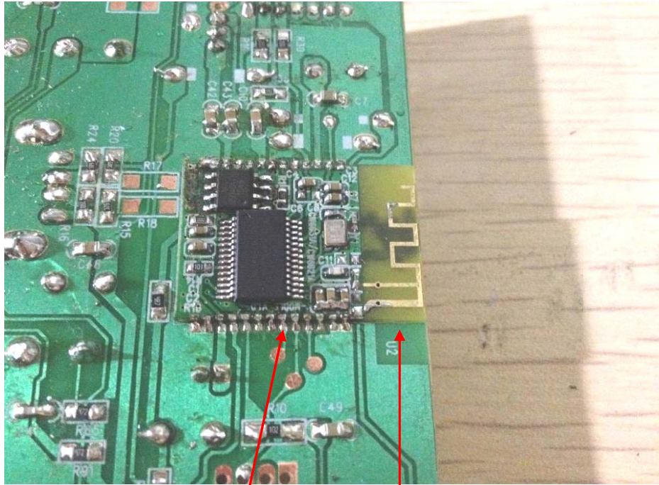
BT Module
