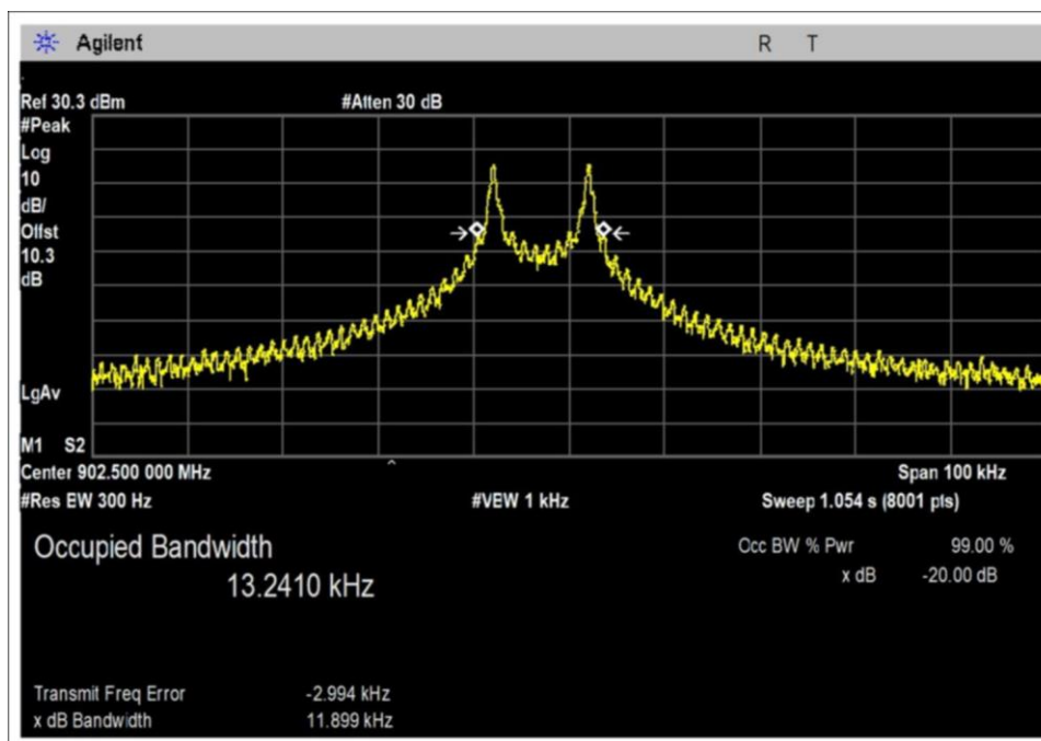
Rate0-01-PWR31-Radio1-Low Channel
