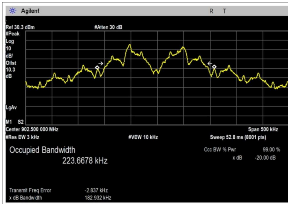
Rate6-01-PWR31-Radio1-Low Channel
