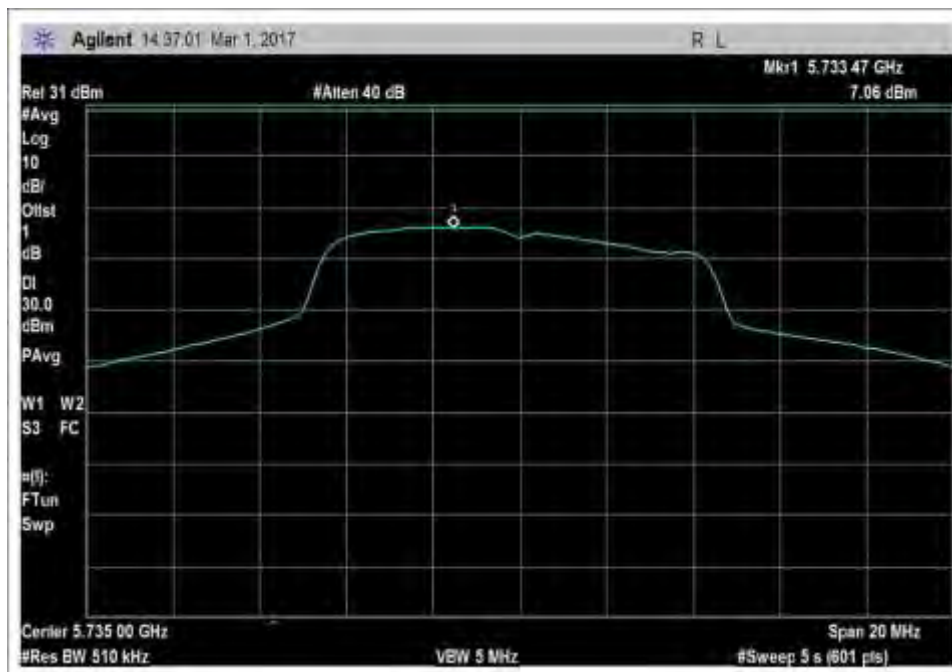
PSD_TX20dBm_5735MHz_chain 1_RMS
