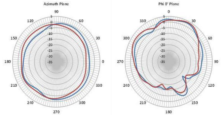
2170 MHz
