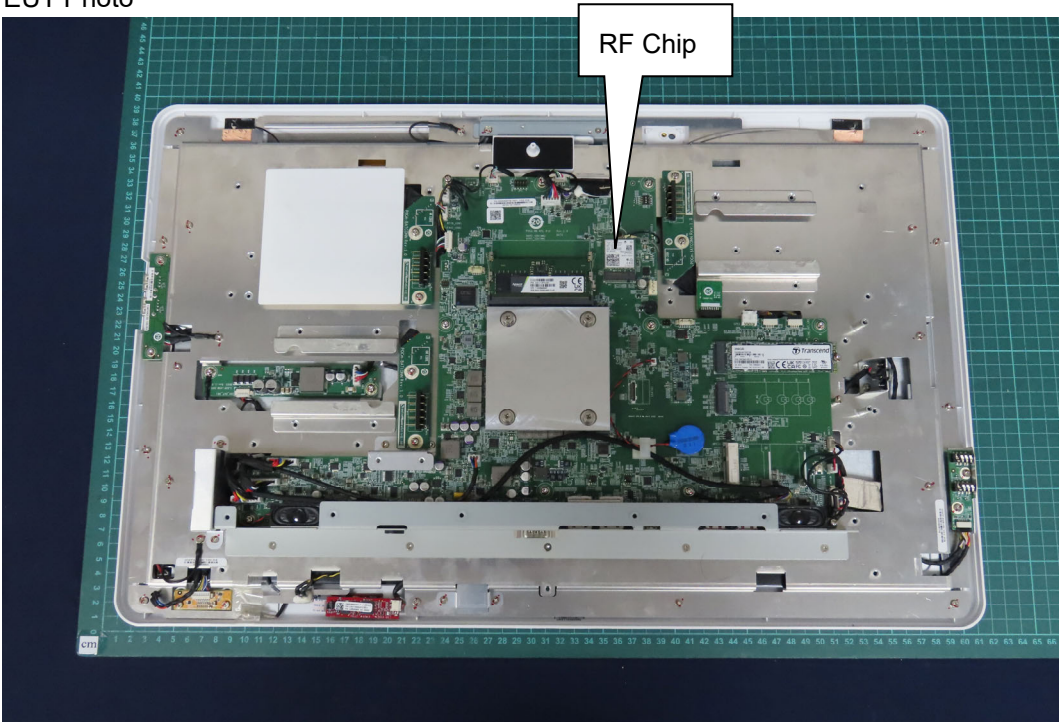
(8) EUT Photo
